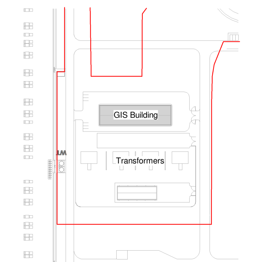
KEYPLAN N.T.S.
